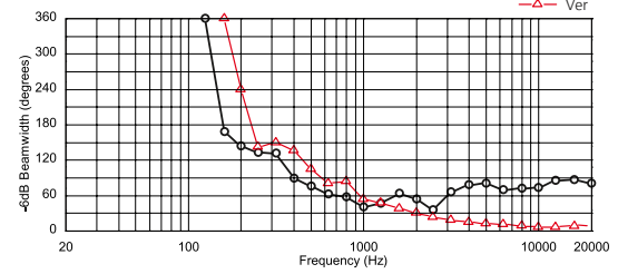
Beamwidth
