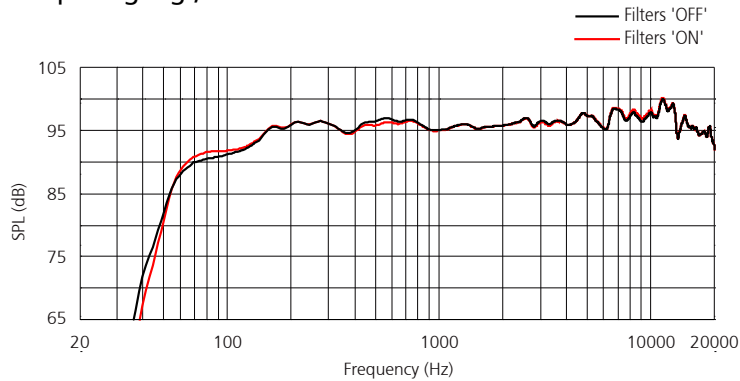
Frequenzgang ‚on axis‘
