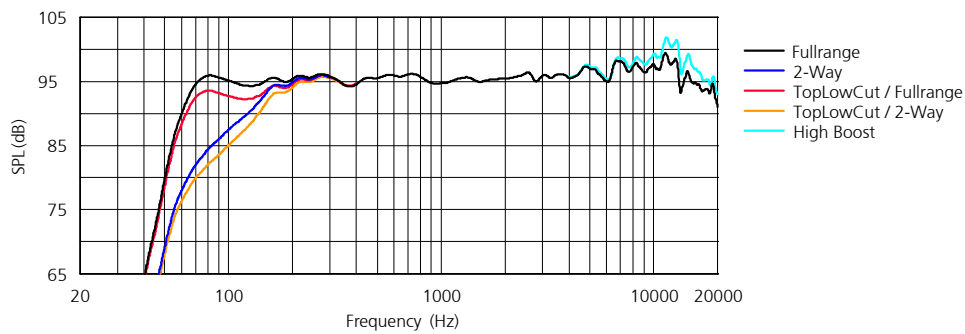
Frequenzgang ‚on axis‘ mit K&F Systemcontroller (Filters ‚OFF‘)
