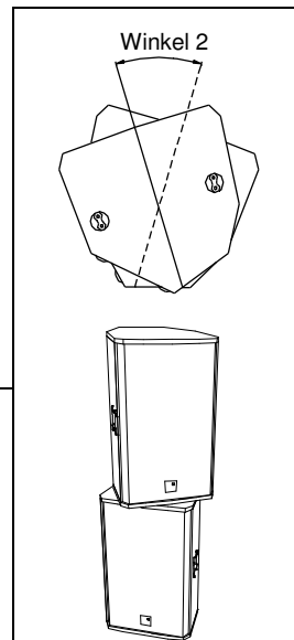
Aufrecht Stehender Lautsprecher
