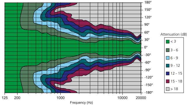
Horizontales Abstrahlverhalten
