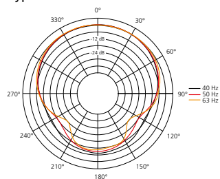
Hyperkardioid
